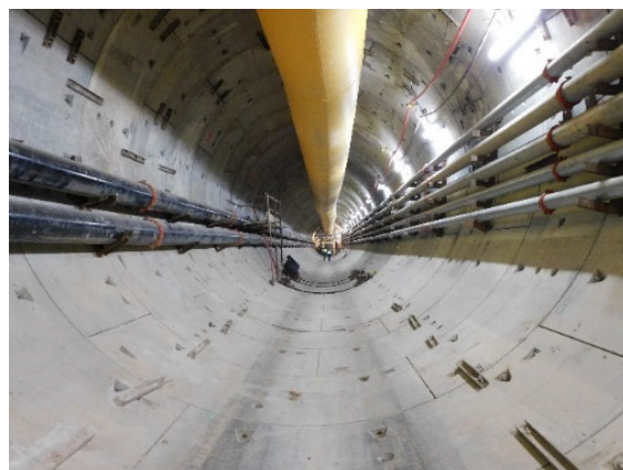
カイロメトロ4号線 トンネル区間
