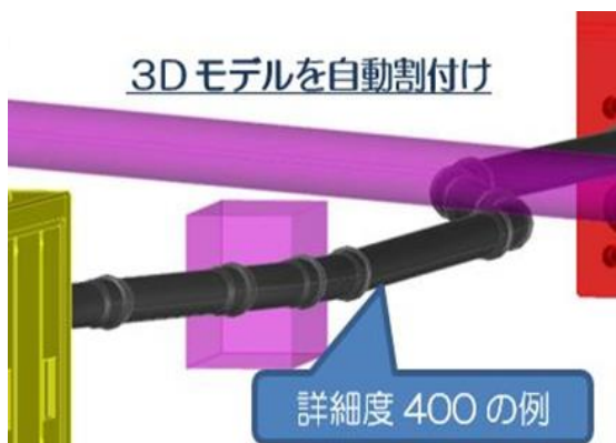
電線共同溝 3D 自動設計システム
