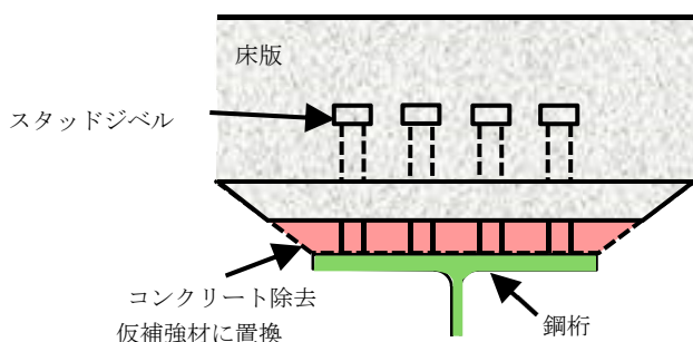
図-1 : コンクリートの除去範囲
