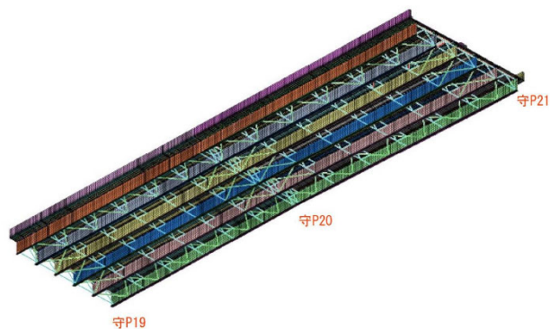
図-2 : FEM モデル (全橋モデル)
